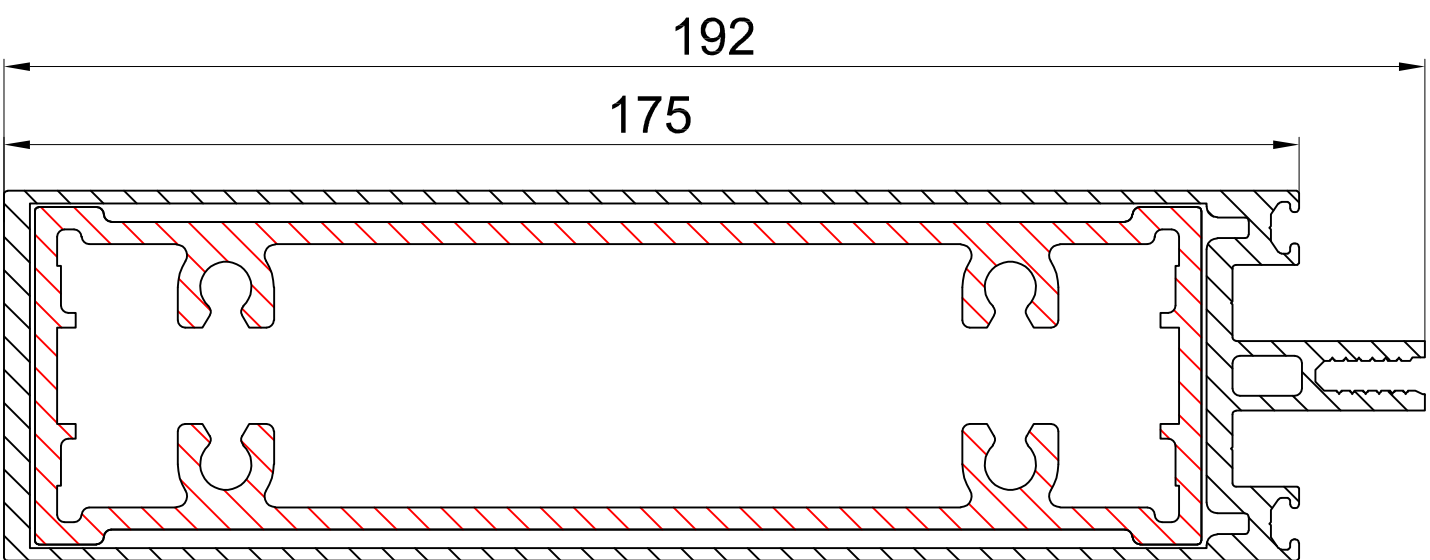
M70034+M70118 Ix=1003cm 4
