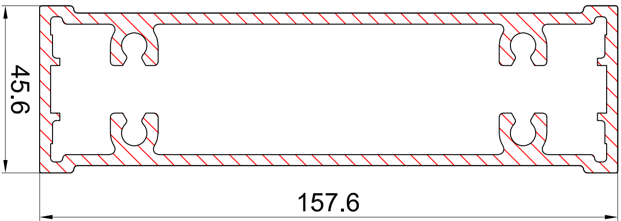
M70118 4320gr/m Ix=470cm 4
